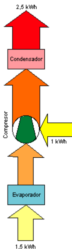
Eficiencia de una bomba de calor
