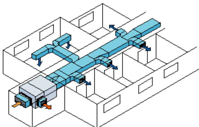
Equipo compacto individual
