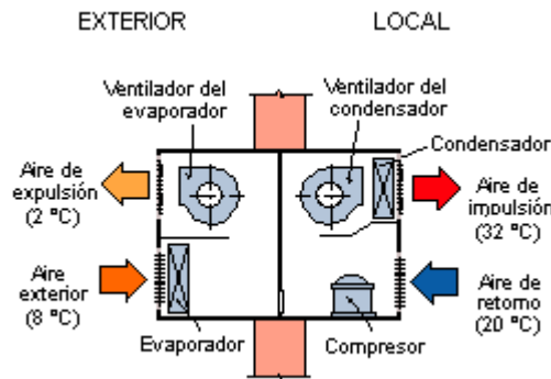
Equipo acondicionador operando como bomba de calor
