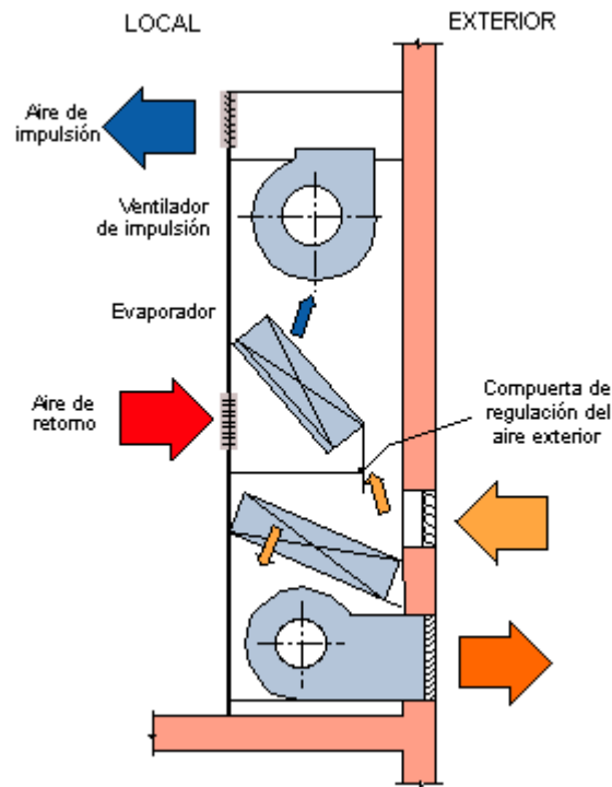
Equipo acondicionador
