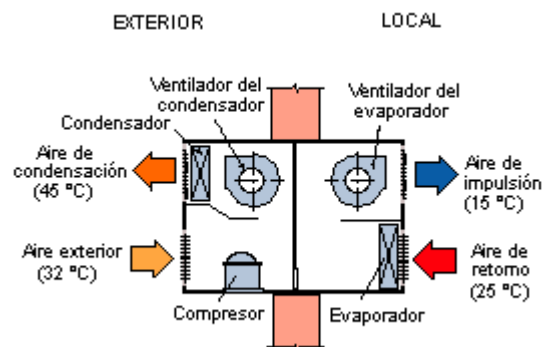
Equipo acondicionador operando en régimen de verano
