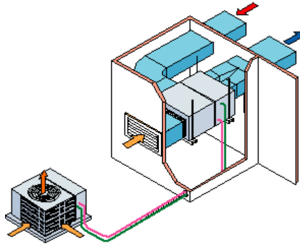
Equipo partido individual
