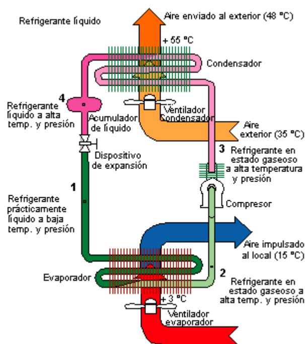
Esquema del circuito frigorífico
